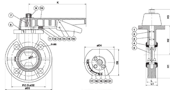
DN50~DN200
